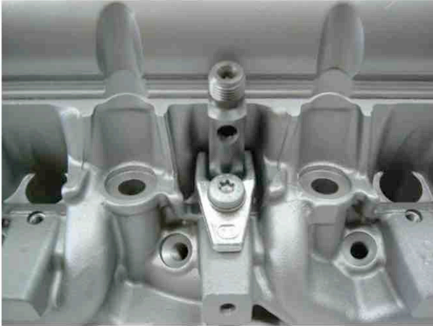
Flachflansch
